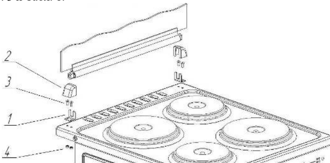
Рис. 3. Установка стеклянной крышки стола.
