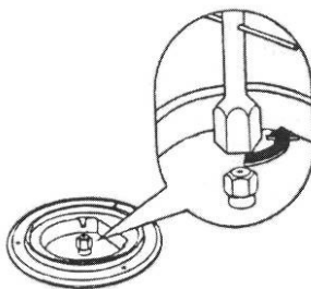
Рис. 8. Замена сопла горелки верхнего стола с помощью ключа 7 мм.
